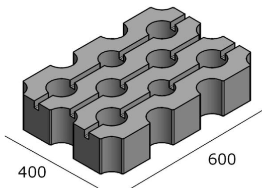
Grasbetontegel HV
